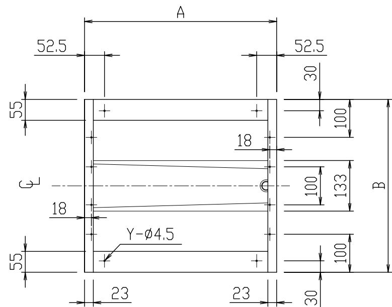
平面図
