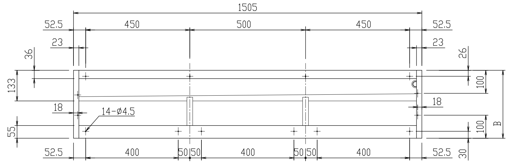
平面図
