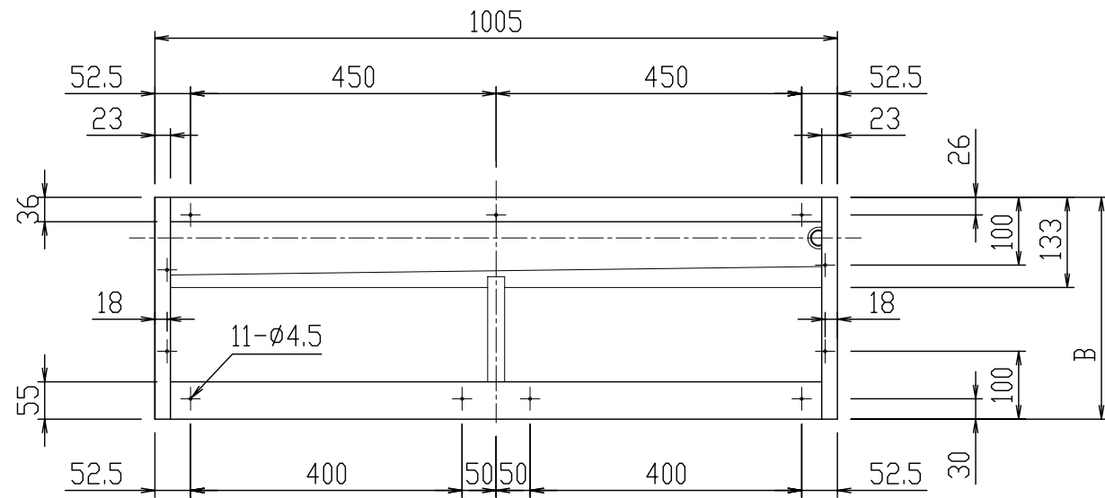
平面図
