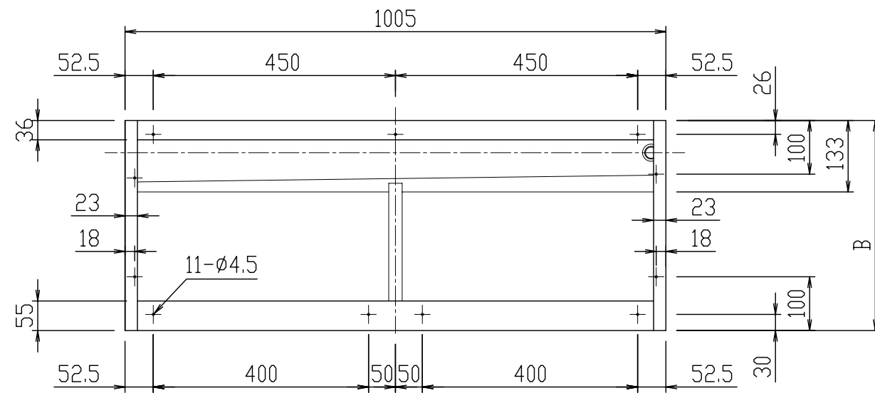
平面図
