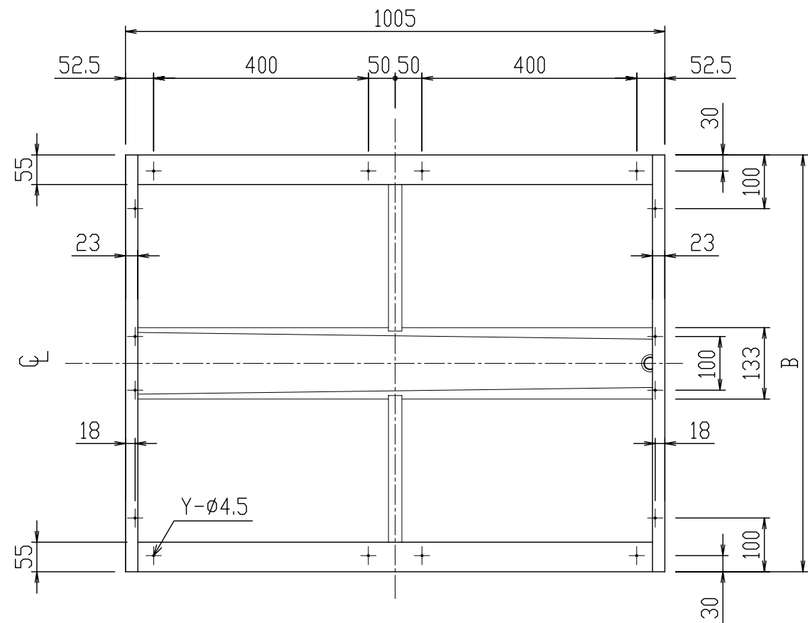
平面図
