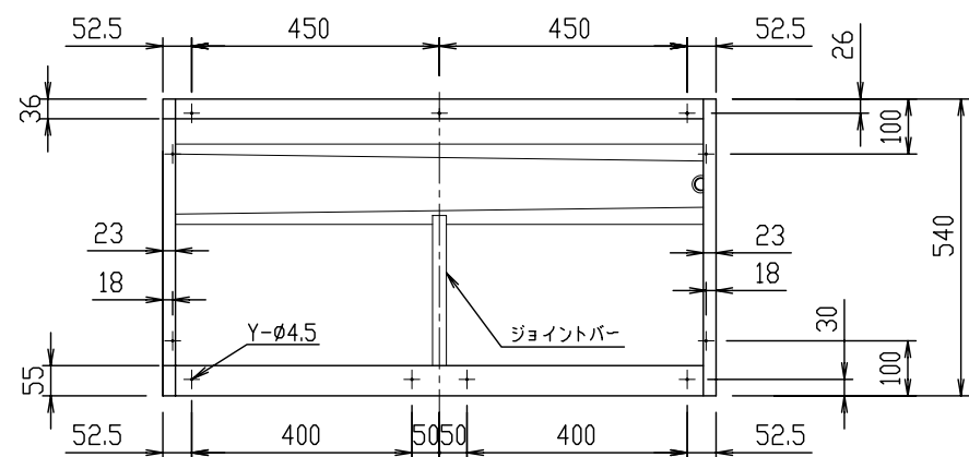
平面図
