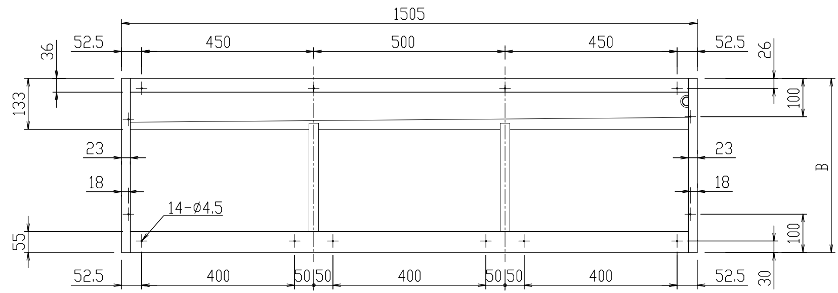
平面図
